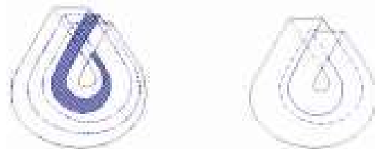
Bande enveloppante et bande de Mœbius dans le cas du huit intérieur
